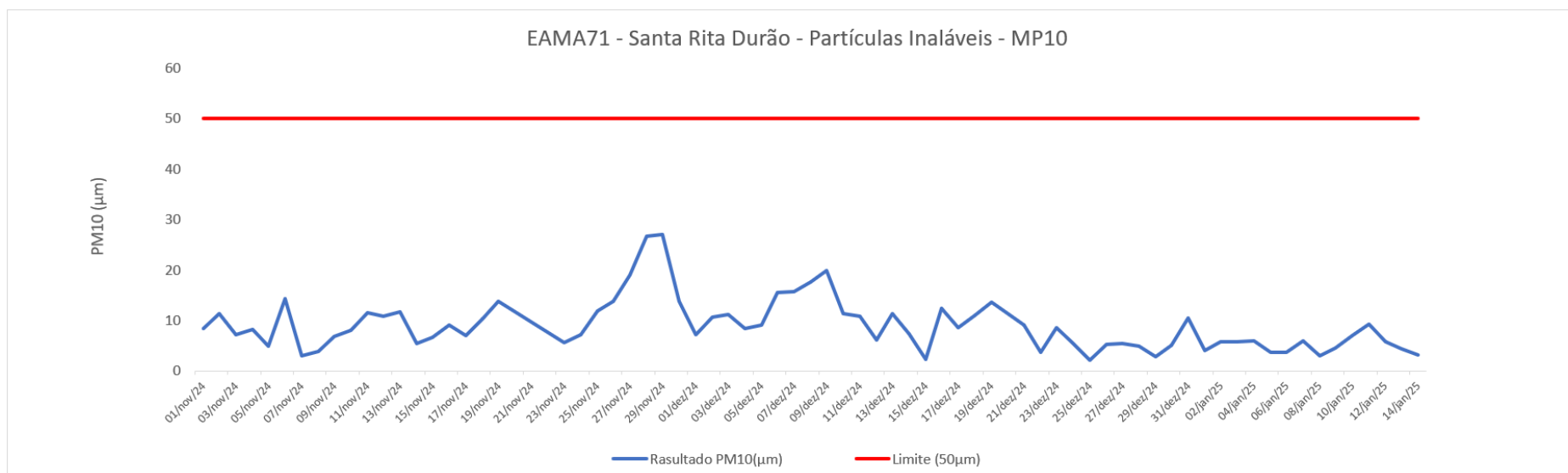
Figura 41 - Resultado de monitoramento do ar, parâmetro PM10, por estação automática EAMA71 entre novembro de 2024 a janeiro de 2025. Fonte: Vale, 2025.
