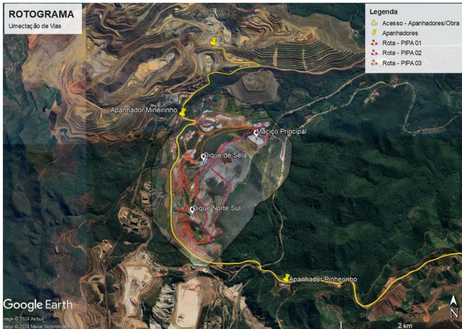
Figura 37 - Rotograma atualizado dos caminhões pipa. Fonte: Vale, 2025.
