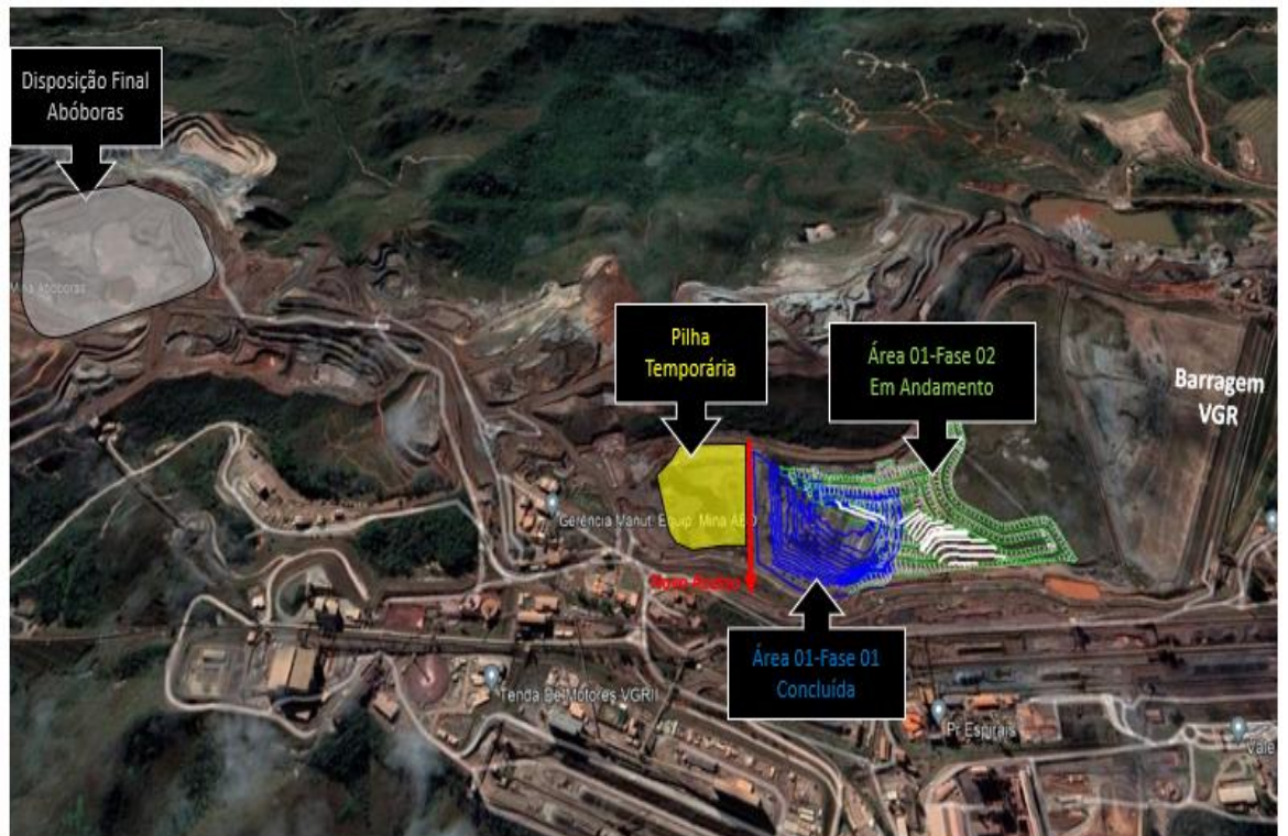
Figura 1 – Vista dos projetos das obras de melhorias na estrutura
