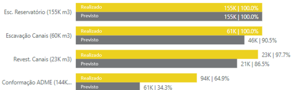
Figura 1 – Avanço da remoção de rejeitos na descaracterização, corte julho/22. Fonte: Vale, 2022.
